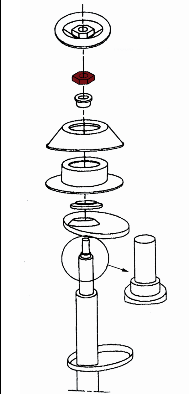
Neue Montage / New Assembly / Nouveau Montage / Montaje nuevo / التركيب الجديد
