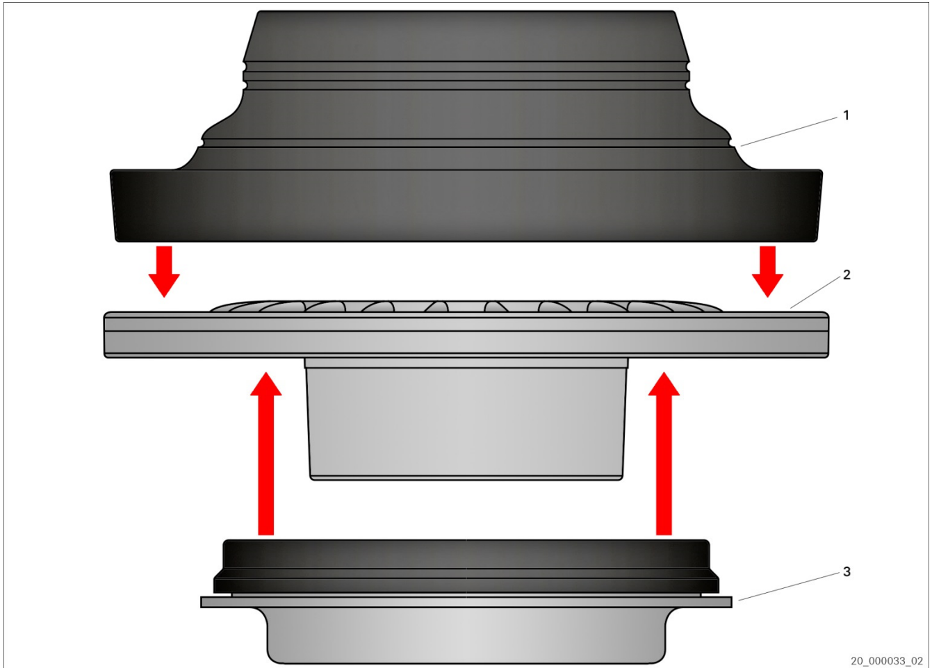
Фиг. 1: Сглобяване на опорния лагер на стойката на амортисьора (пример)
