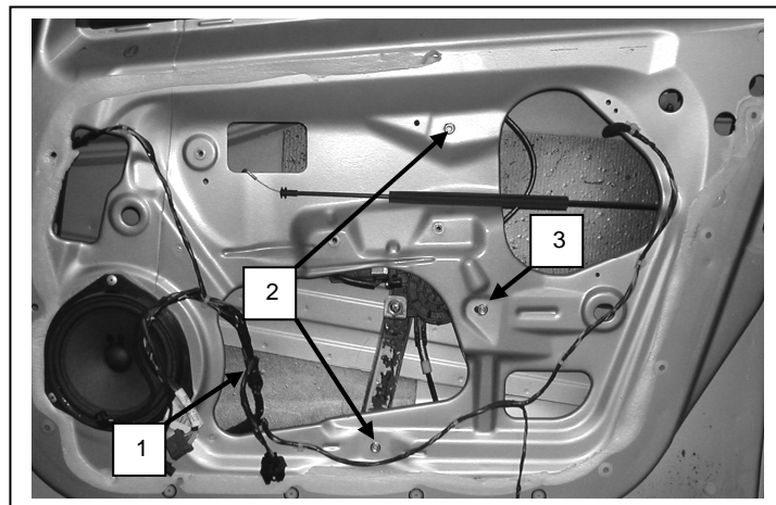
Porta lato destro, Portière avant droite, Right front door, Puerta lado derecho, Vorne rechte Tür, Porta frente dirieta, Sag on kapı, πόρτα εμπρόςθια δεξιά
