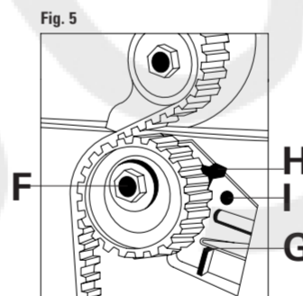
FIGURA 5 Allentare il bullone di bloccaggio F, agendo nel punto indicato, G, del tenditore automatico; portare l'indicatore mobile, H, nella posizione di massima tensione, e, dopo aver fatto coincidere il punto H con il Punto I, serrare il bullone di bloccaggio F.
