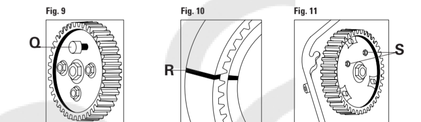
FIGURA 9 Insertar la herramienta específica de inmovilización de la polea de bomba de inyección "O". FIGURA 10 Verificar la correcta alineación de las marcas de puesta a punto "R". FIGURA 11 Insertar las herramientas específicas para inmovilizar la polea de la bomba de inyección "S". FIGURE 9 Introduire l'outil approprié de blocage poulie pompe d'injection O. FIGURE 10 Contrôler le correct alignement des points de repère de phase R. FIGURE 11 Introduire les outils appropriés de blocage poulie pompe d'injection S.
