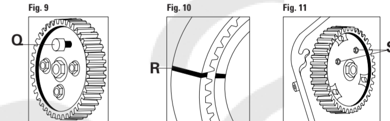
FIGURA 9 Inserire l'apposito attrezzo di bloccaggio della puleggia della pompa di iniezione Q.
