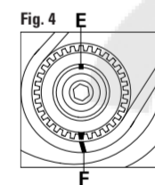
FIGURA 4 Controllare il corretto allineamento delle tacche di fase E ed F.
