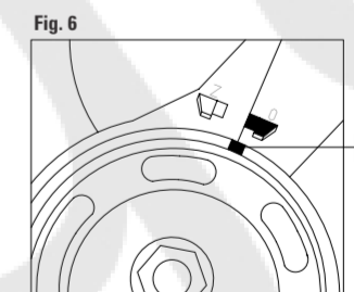
FIGURA 5 Controllare il corretto allineamento della tacca di fase D. FIGURA 6 Controllare il corretto allineamento della tacca di fase P.
