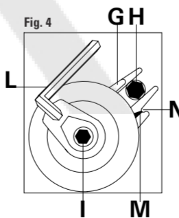
FIGURA 4 Asegurarse que la lamina C esta fijada por debajo del tornillo de fijación H. Luego aflojar el tornillo de fijación I, y girar el tensor de la correa en sentido de las agujas del reloj actuando con la llave L sobre el excéntrico de regulación hasta lograr la alineación de la marca M con la muesca N. Por último, apretar el tornillo de fijación I.
