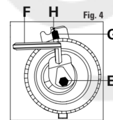
FIGURA 4 Aflojar el tornillo de fijación E del tensor de correa. Actuando con la llave hexagonal F sobre el excéntrico de regulación, girar el tensor de la correa en sentido de las agujas del reloj hasta que el indicador G y la marca H estén alineados. Por último, apriete el tornillo de fijación del tensor.
