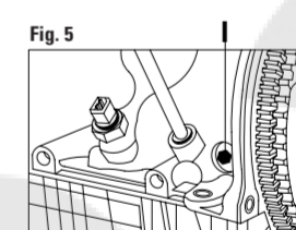
FIGURA 5 Togliere il tappo cieco I dal blocco cilindri.
