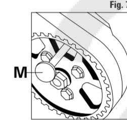
FIGURA 7 Insertar la herramienta específica para inmovilizar la bomba de inyección M.
