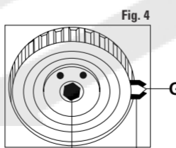
FIGURA 2 Aflojar el tornillo de fijación B, girar el tensor de correa sobre el excéntrico en sentido de las agujas del reloj, utilizando la llave de regulación C. FIGURA 3 Alinear el indicador D del tensor de la correa con la muesca E. Finalmente, apretar el tornillo de fijación B. FIGURA 4 Aflojar el tornillo de fijación F del tensor de correa. Girar el tensor de correa en sentido de las agujas del reloj hasta alinear la marca G con la zona de control H.
