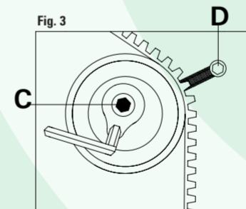
FIGURA 3 Aflojar el tornillo de fijación C. Suelte el tensor de correa hasta la obtención de la tensión correcta. Apretar el tornillo de fijación C. Asegurarse que el resorte D quede insertado con su respectivo tornillo de fijación.
