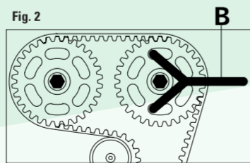
FIGURA 1 Inserire l'apposito attrezzo di bloccaggio dell'albero a camme A. FIGURA 2 Inserire l'apposito attrezzo di bloccaggio B, per mantenere gli ingranaggi in tensione.
