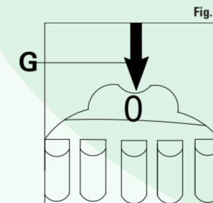
FIGURA 4 Marcas de referencia sobre el volante de inercia del motor; Verificar la correcta alineación de las marcas de fase F. FIGURA 5 Marcas de referencia sobre el volante de inercia del motor; Verificar la correcta alineación de las marcas de fase G.
