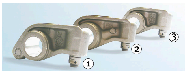
Фигура 1: Преглед на трите различни вида кобилицы
