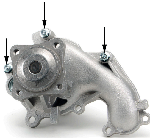
Снимка 2: Модифицирани точки за монтиране на помпата за охлаждаща течност
