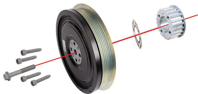
Снимка 2: Болтове на разединителя на ремъчната шайба, централния болт на колянния вал, разединителя на ремъчната шайба и шайбата с диамантено покритие
