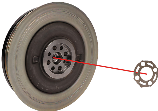
Снимка 1: Страна на колянния вал на разединителя на ремъчната шайба с диамантено покритие. В посочените по-горе комплекти, шайбата с диамантено покритие вече е поставена в положението за монтаж на разединителя на ремъчната шайба
