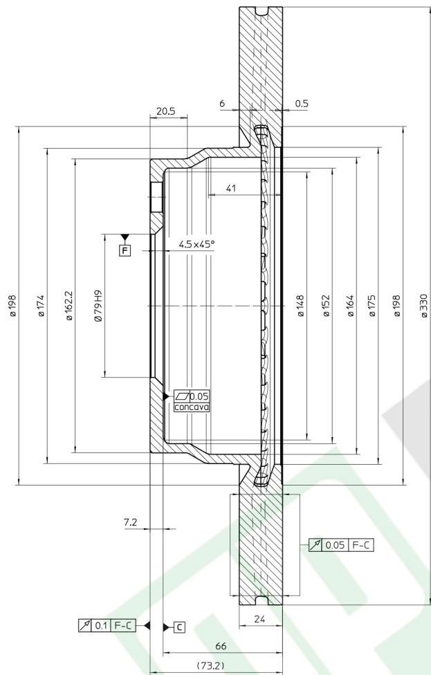
Sezione A-A
