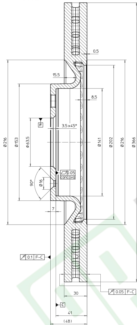
Sezione A-A
