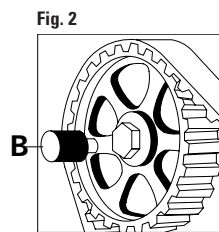
FIGURA 1 Controllare il corretto allineamento delle tacche di fase A. FIGURA 2 Inserire l'apposito attrezzo di bloccaggio dell'albero a camme B.
