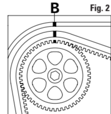
FIGURA 1 Verificar que la marca de puesta a tiempo este en línea con la marca del cárter de la distribución A. FIGURA 2 Verificar la correcta alineación de las marcas de puesta en fase B.
