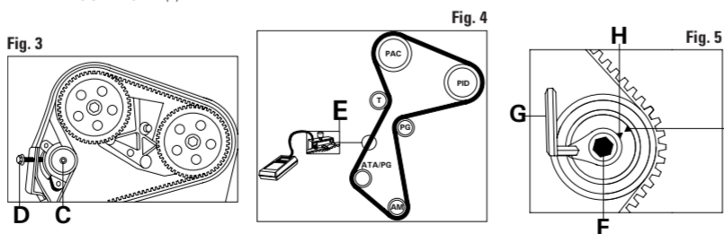
FIGURA 3 Allentare il bullone di bloccaggio C e inserire l'apposito attrezzo di tensionamento D, avvitandolo fino alla corretta tensione; serrare quindi il bullone di bloccaggio C. FIGURA 4 Inserire l'apposito attrezzo di misura del tensionamento E, nel punto indicato, ed agire sul tendicinghia fino ad un valore compreso tra 42.3 e 51.7 unità SEEM (per modello Renault Kangoo); 37 unità SEEM (per modello Renault Espace); 61 ± 5 Hz (per modello Volvo S40). FIGURA 5 Allentare il bullone di bloccaggio F e ruotare in senso antiorario il tendicinghia utilizzando la chiave esagonale G, fino ad allineare le tacche di fase H ed I; serrare, quindi, il bullone di bloccaggio F.
