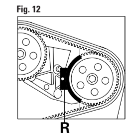
FIGURA 11 Verificar la correcta alineación de las marcas de fase Q. FIGURA 12 Insertar la herramienta para inmovilización de polea de bomba de inyección R.
