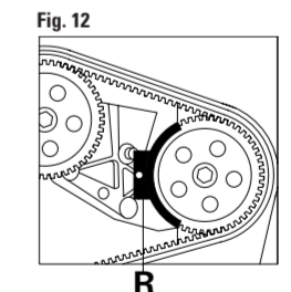
FIGURA 11 Controllare il corretto allineamento delle tacche di fase Q. FIGURA 12 Inserire l'apposito attrezzo di bloccaggio della puleggia della pompa di iniezione R.
