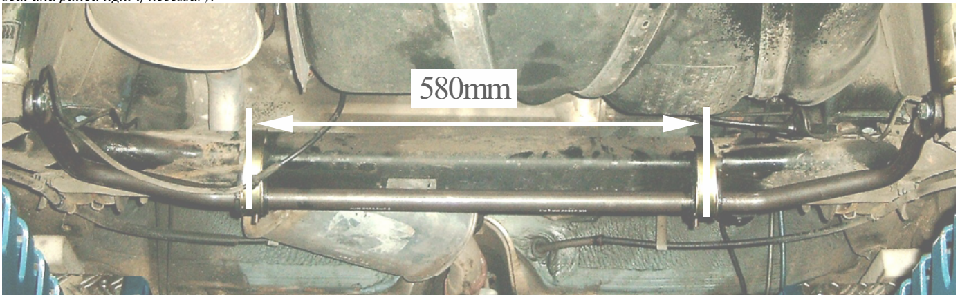
Abbildung/figure 5: Abstand der Lager
