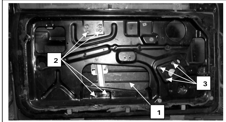
Puerta lado izquierdo, Left rear door
