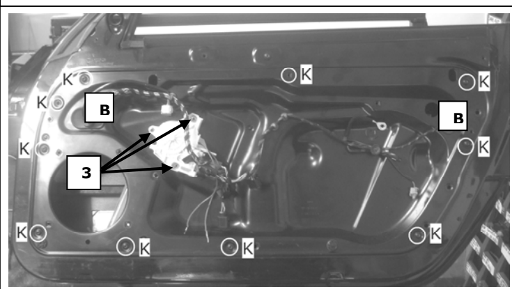
Porta lato destro, Portière avant droite, Right front door, Puerta lado derecho, Vorne rechte Tür, Porta frente diarieta, Sag on kapi, πόρτα εμπρόςθια δεξιά
