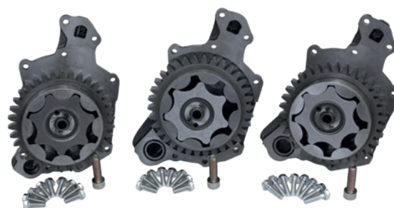
MAN 油泵
