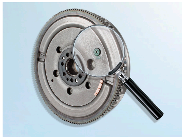
Obrázek 1: 415 0142 10 – transportní pojistka zůstává v dvouhmotovém setrvačnicku
