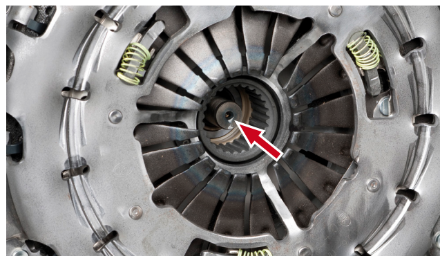
Billede 2: 415 0377 10 med en påmonteret kobling (SAC)
