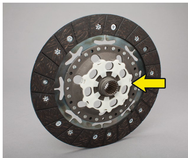
Bild 1: LuK kopplingslamell med plastbricka
