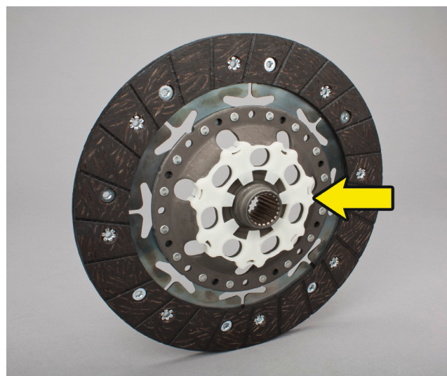
Зображення 1: Диск зчеплення LuK з пластмасовим кільцем
