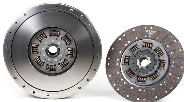
Εικόνα 2: Διπλός συμπλέκτης LuK με ίδια κέντρα
