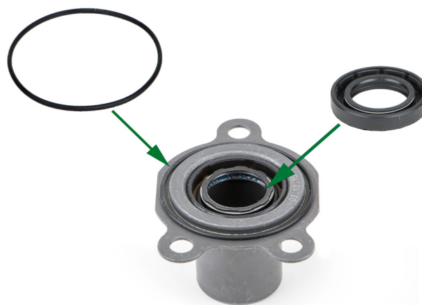
Manșon de ghidare cu garnitură O-ring și garnitură pentru arbore deja montate
