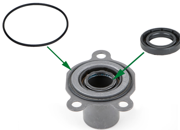
Зображення 1: Направляюча втулка з попередньо встановленим ущільнювальним кільцем і сальником вала
