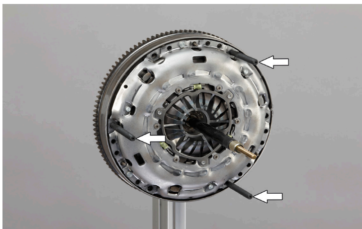
Slika 2: Svorni vijci za prihvat SAC alata – označeni bijelim strelicama
