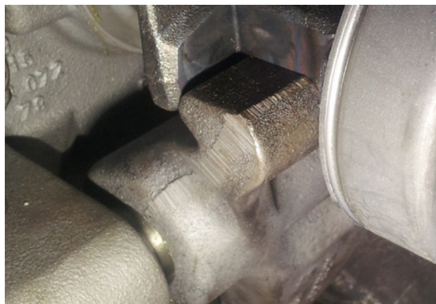
Bild 2: Ausrückgabel mit abgerundeter Nockenform
