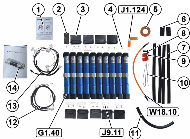
Abbildung 1 HV- Batterie Reparaturset Kit - Lieferumfang
