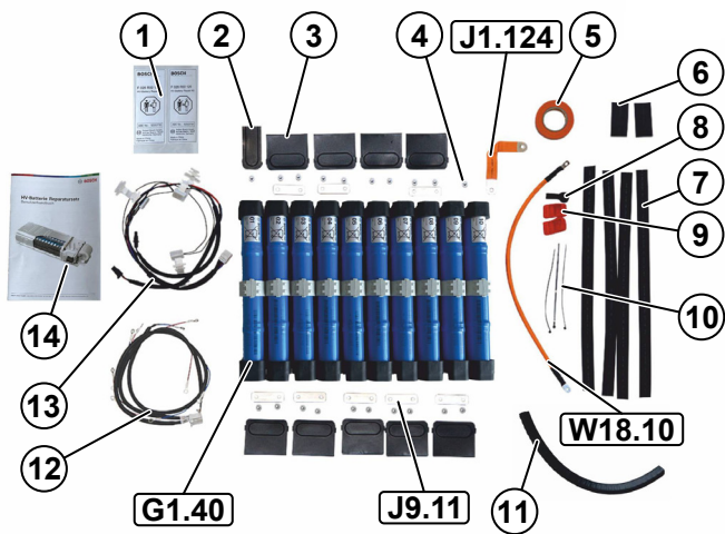
Afbeelding 1 HV-accureparatieset - leveringsomvang
