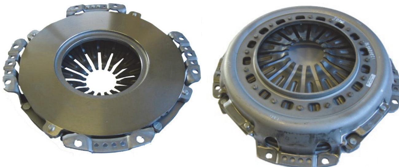
Abb. 1: 330 mm Einfach-Membranfederkupplung
