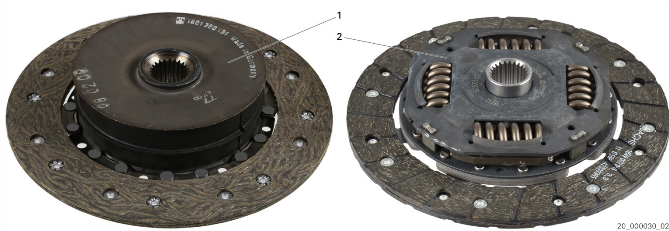
Obr. 1: Spojkové kotúče Porsche
