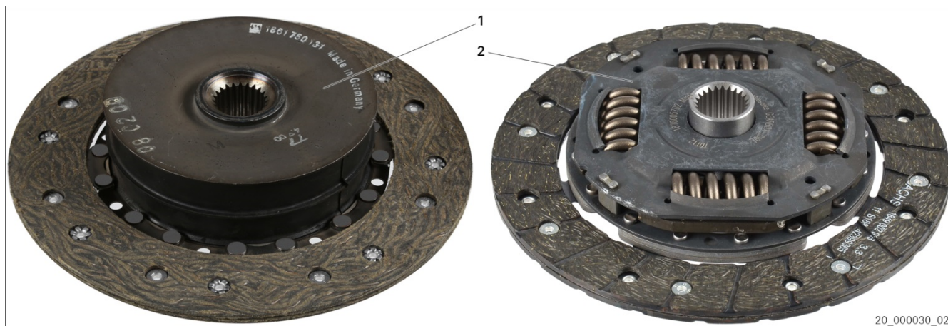
Εικ. 1: Δίσκοι συμπλέκτη Porsche
