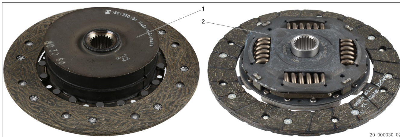
Sl. 1: Diskovi kvačila, Porsche
