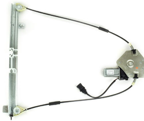
Nuestro Elevallunas / Our window regulator / Notre lève-vitre / Nosso elevador de vidro
