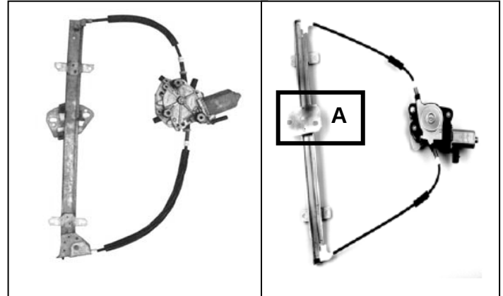
Elevalunas original – lève-vitre original Nuestro elevalunas – notre lève-vitre – oem window regulator – levandator – our window regulator – nosso de vidro original levantador de vidro
