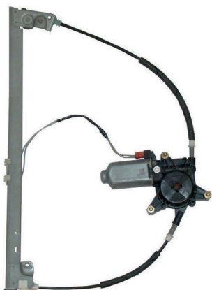
Elevallunas original / OEM window regulator / Lève-vitre original / Elevador de vidro original
