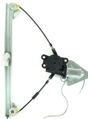
Nuestro Elevallunas / Our window regulator / Notre lève-vitre / Nosso elevador de vidro
