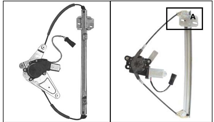
Elevalunas original – lève-vitre original Nuestro elevallunas – notre lève-vitre – oem window regulator – levandator – our window regulator – nosso de vidro original levantador de vidro
