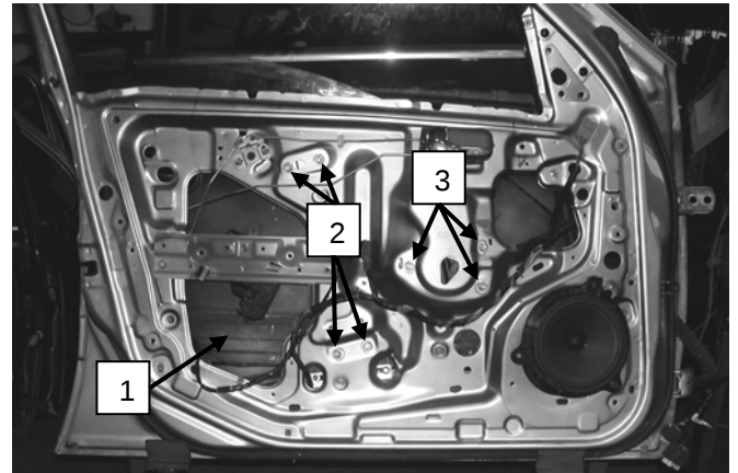
Puerta lado izquierdo, Portière arrière gauche, Left rear door, Porta traseira esquerda
