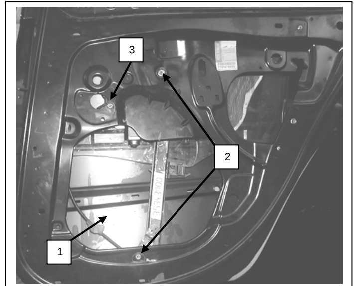
Puerta lado derecho, Portière avant droite, Right front door, Porta frente diresa,
