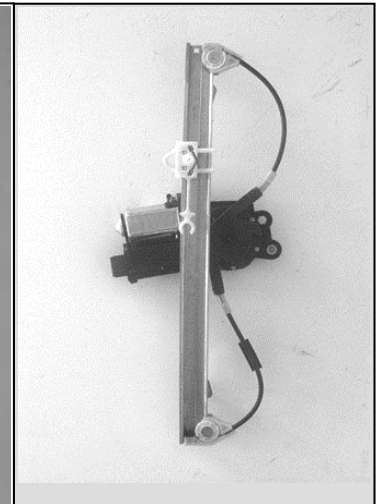
Nuestro elevavinas – notre lève-vitre – our window regulator – nosso levantador de vidro
