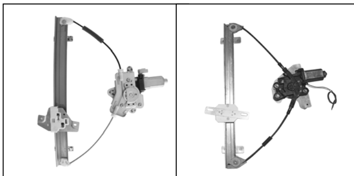
Elevallunas original – lève-vitre original Nuestro elevallunas – notre lève-vitre – oem window regulator – levandator – our window regulator – nosso de vidro original levantador de vidro
