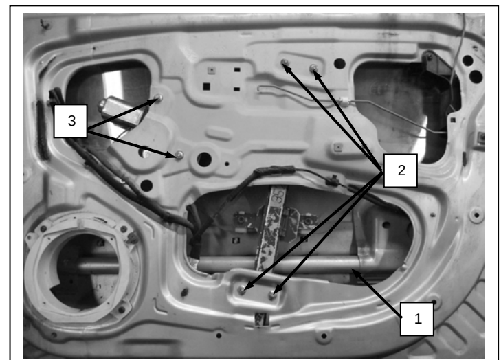
Puerta lado derecho, Portière avant droite, Right front door, Porta frente direita
