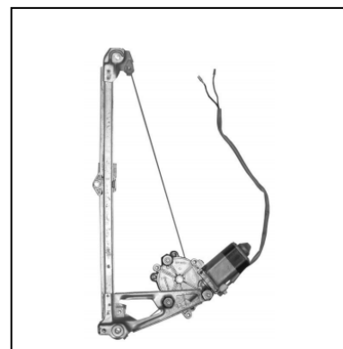
nuestro elevavinas – our window regulator – notre lève-vitre – nosso levantador de vidro
