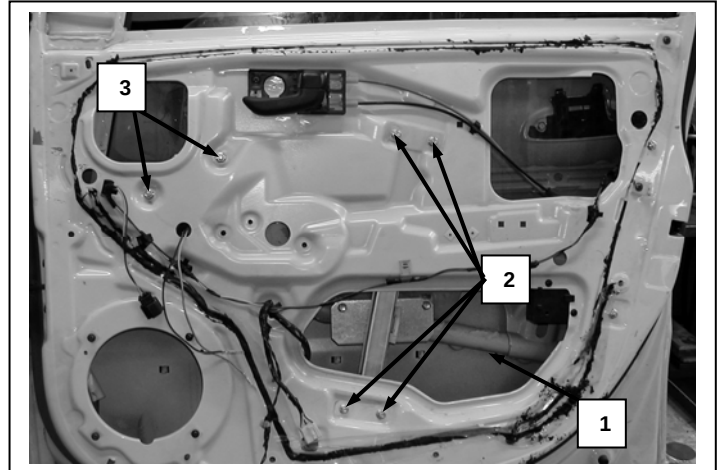
Puerta lado derecho, Portière avant droite, Right front door, Porta frente diresa
