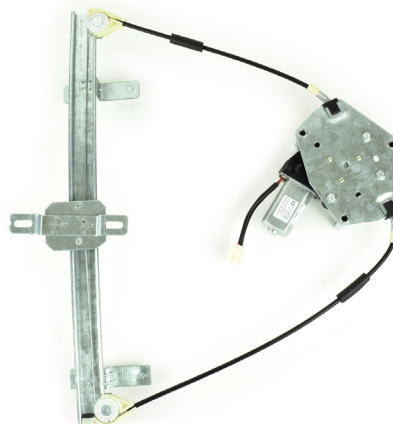
Nuestro Elevallunas / Our window regulator / Notre lève-vitre / Nosso elevador de vidro
