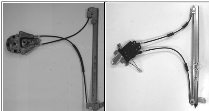
Elevalunas original – lève-vitre original Nuestro elevallunas – notre lève-vitre – oem window regulator – levandator – our window regulator – nosso de vidro original levantador de vidro
