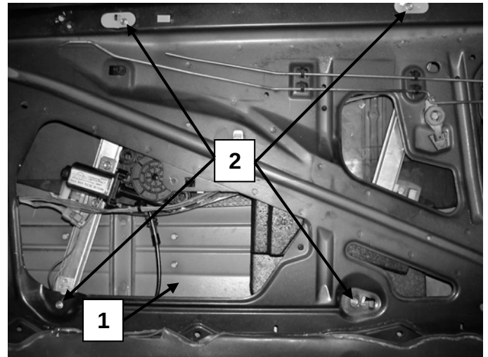
Puerta lado derecho, Portière avant droite, Right front door, Porta frente direita
