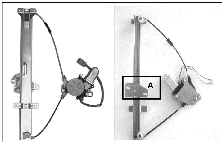
Elevavinas original – lève-vitre original Nuestro elevavinas – our window – oem window regulator – levandator regulator – notre lève-vitre – nosso de vidro original levantador de vidro
