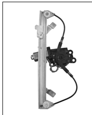
Nuestro elevallunas – notre lève-vitre – our window regulator – nosso levantador de vidro
